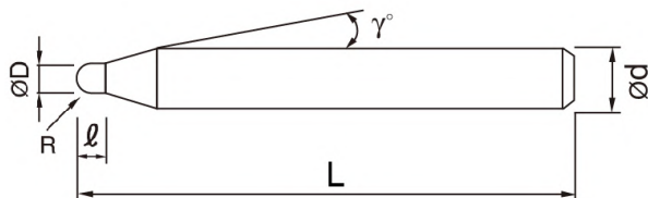
形式 I：全刀長型
