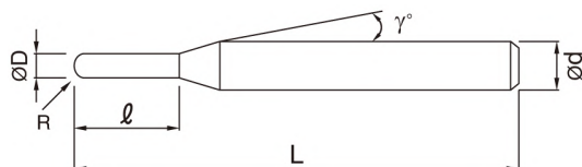
形式 I：全刀長型
