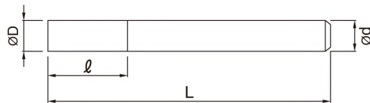
形式 I：全刃長型
