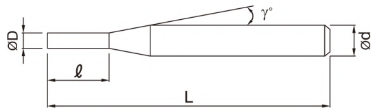
形式 I：全刃長型
