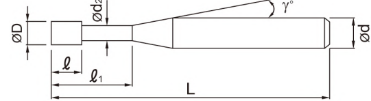
形式 II：深溝型
