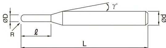
形式 I：全刀長型
