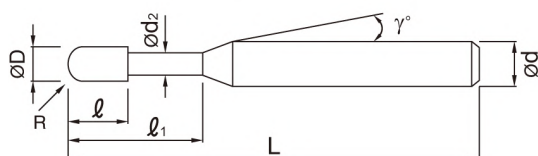
形式 II：深溝型
