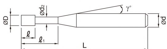
形式 II：深溝型
